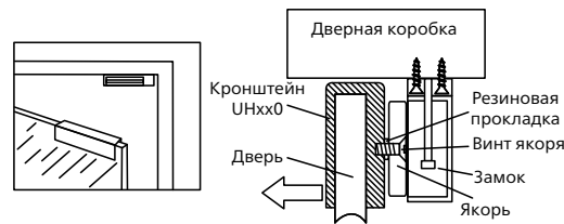
Рис.4 Монтаж на стеклянную дверь с помощью кронштейна U типа (UHxx0).
