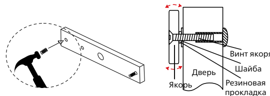
Рис.7 Установка фиксирующих штифтов
