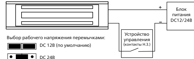
Рис.10 Схема подключения DL280 и DL350.
