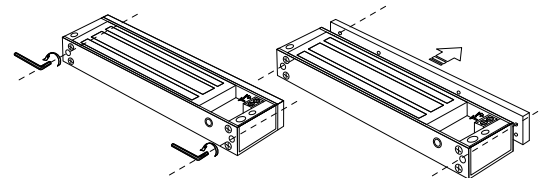
Рис.6 Съём крепёжной панели.
