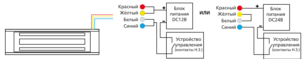
Рис.9 Схема подключения DL180.
