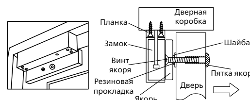
Рис.1 Стандартный монтаж на дверную коробку.
