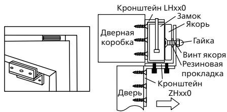
Рис.3 Монтаж с помощью кронштейнов L и Z типов (LHxx0, ZHxx0).
