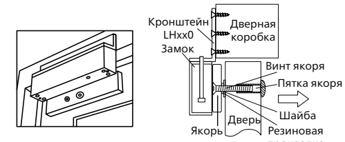
Рис.2 Монтаж с помощью кронштейна L типа (LHxx0).
