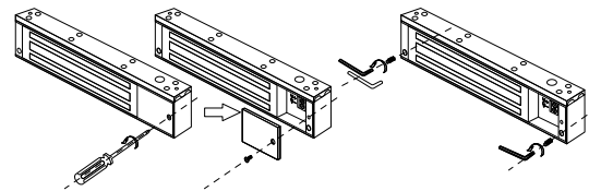
Рис.5 Удаление защитных болтов для замков DL280 и DL350.
