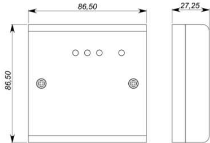
Рис 7а. Габаритные размеры, модификация 1
