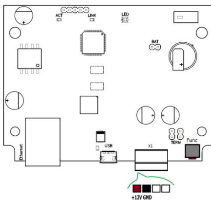
Рис. 2б. Внешний вид платы контроллера модификации 2
