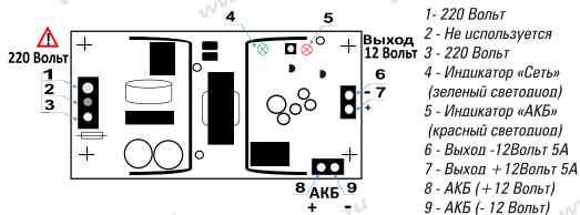
Рис.1 Схема электрической монтажной
