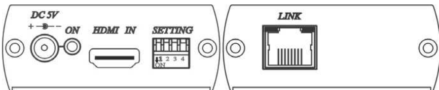
Рис.5 Панель подключения HE01ST
