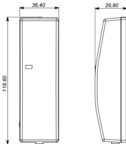
Рис 8. Габаритные размеры
