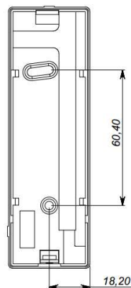
Рис 9. Разметка крепежных отверстий
