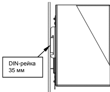
Рисунок 2 — Размещение изделия на DIN-рейке
