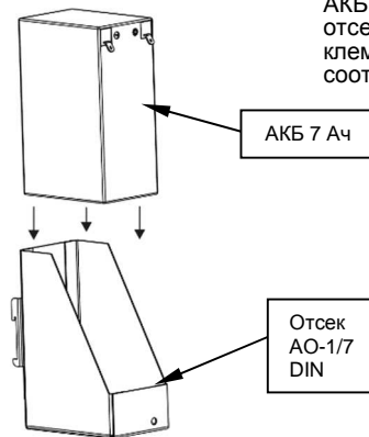
Рисунок 1 — Общий вид изделия с установкой АКБ
