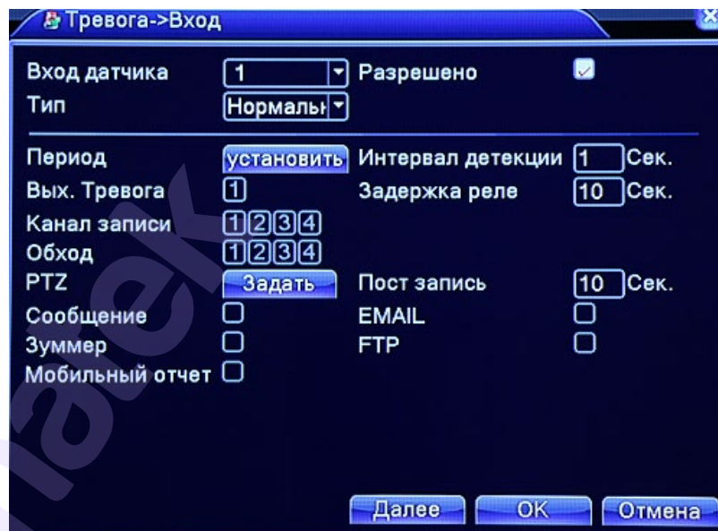
Рис. 4.49 Настройки входов тревоги
