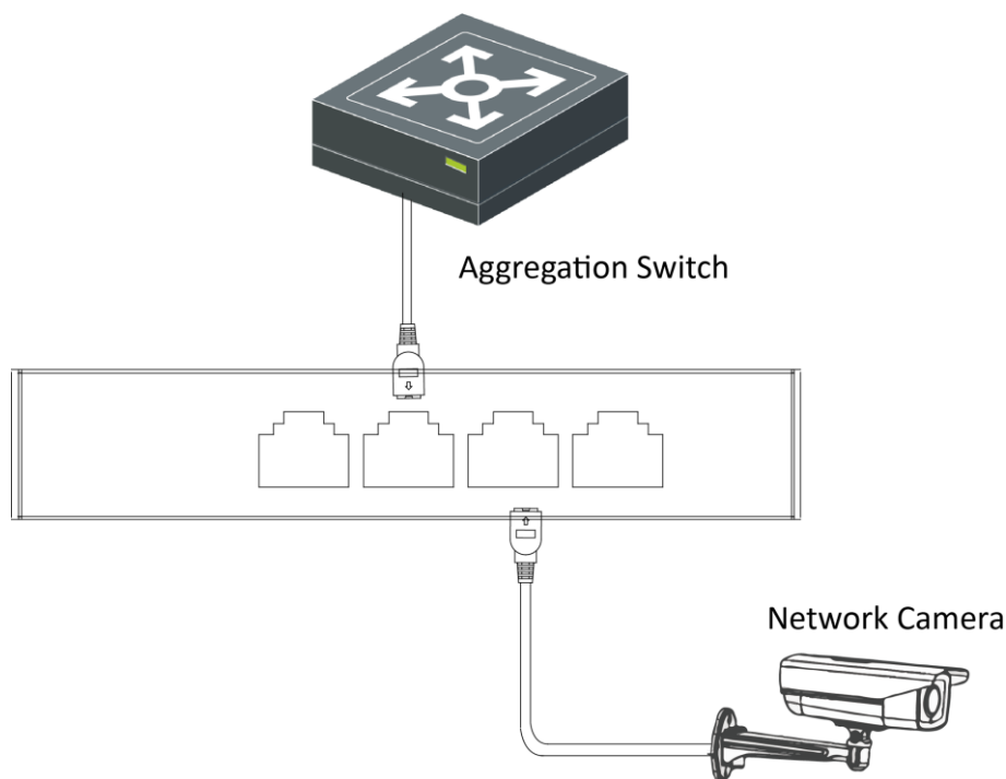
Рисунок 3-3 Подключение к RJ45 портам
