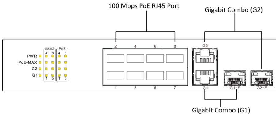
Рисунок 1-1 SWT-1309P
