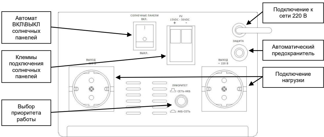
Рисунок 5 – Боковая сторона инвертора Teplocom Solar 800
