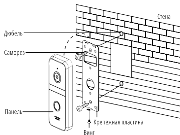
Рис. 9 Фронтальная установка вызывной панели
