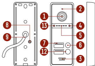
Рис. 5 Вызывная панель FANTASY 2 FHD
