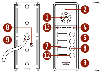
Рис. 6 Вызывная панель FANTASY 4 FHD
