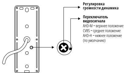
Рис. 8 Регулировка громкости динамика и выбор типа видеосигнала
