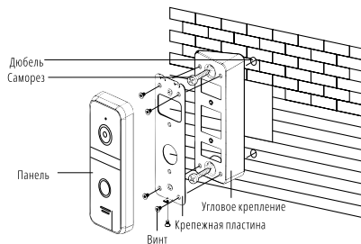
Рис. 10 Установка вызывной панели под углом 30°
