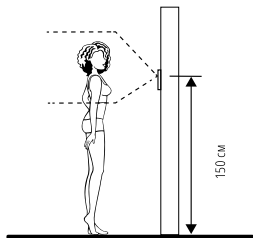
Рис. 7 Рекомендуемая высота установки видеопанели
