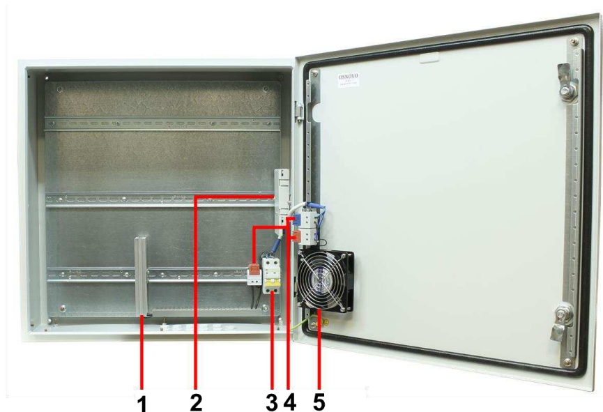
Рис. 8 Уличная станция OS-66T1 с системой обогрева, внутренние элементы
