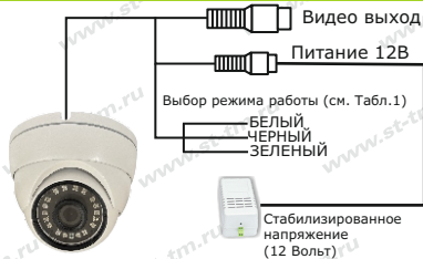
Рис.1 Схема подключения
