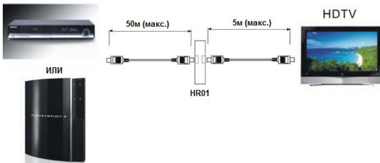
Рис.1 Схема подключения HR01
