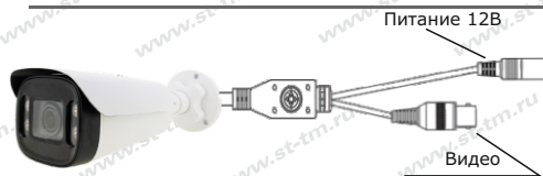
Рис.1 Схема подключения
