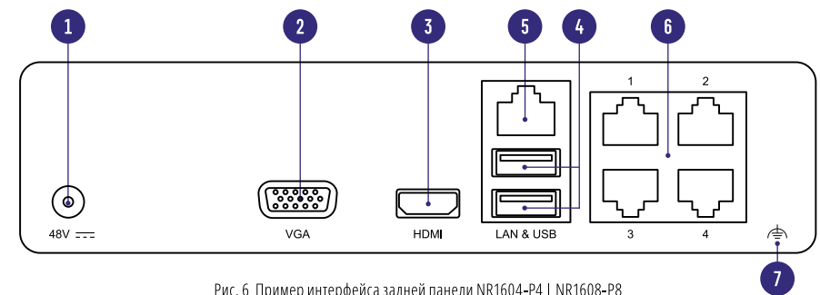
Рис. 6 Пример интерфейса задней панели NR1604-P4 | NR1608-P8
