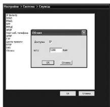
Рис. 15 Служба Облако
