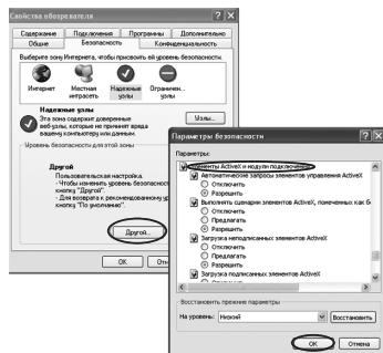
Рис. 12 Настройки браузера
