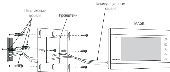
Рис. 5 Монтаж видеодомофона.
