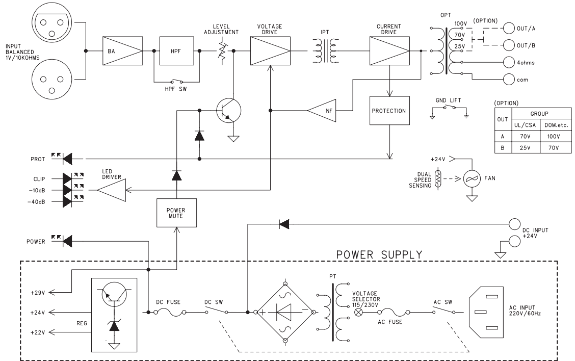
- PA-6324/ 6336/ 6348
