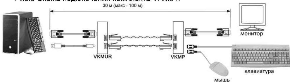
Рис.7 Схема подключения комплекта VKM02.
