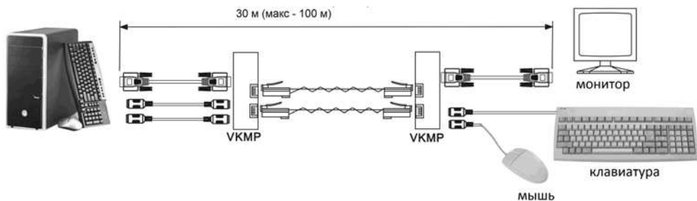
Рис.6 Схема подключения комплекта VKM01.
