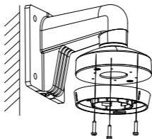
Рисунок 2-14 Крепление монтажной платформы на кронштейне
