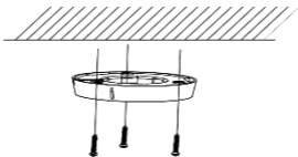
Рисунок 2-4 Крепление монтажной платформы
