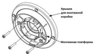
Рисунок 2-8 Крепление монтажной платформы на крышке для монтажной коробки
