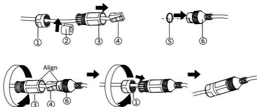
Рисунок 2-15 Установка гермоввода
