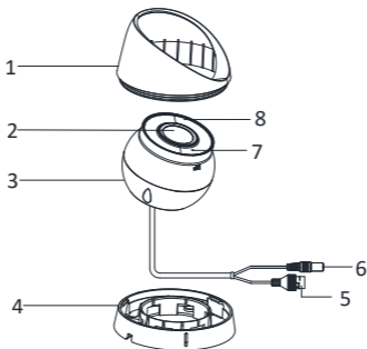
Рисунок 1-4 Камера в корпусе «шар», Тип V
