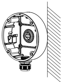
Рисунок 2-9 Крепление корпуса монтажной коробки на потолке/стене
