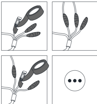
Рисунок 2-16 Герметизация кабелей
