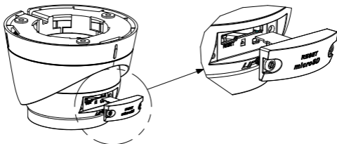
Рисунок 2-1 Демонтаж крышки и установка карты памяти
