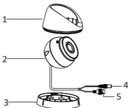
Рисунок 1-3 Камера в корпусе «шар», Тип III/IV
