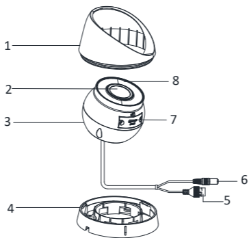
Рисунок 1-5 Камера в корпусе «шар», Тип VI
