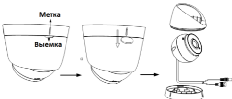
Рисунок 2-3 Разбор камеры
