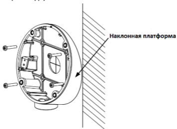
Рисунок 2-12 Крепление наклонной платформы на потолке/стене
