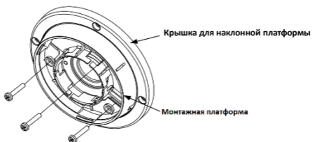
Рисунок 2-11 Крепление монтажной платформы
