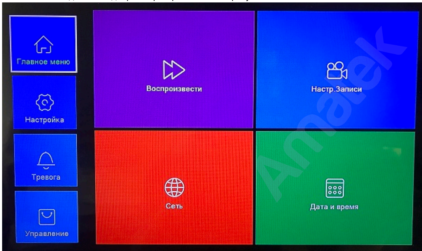
Рис. 4.1 Главное меню
