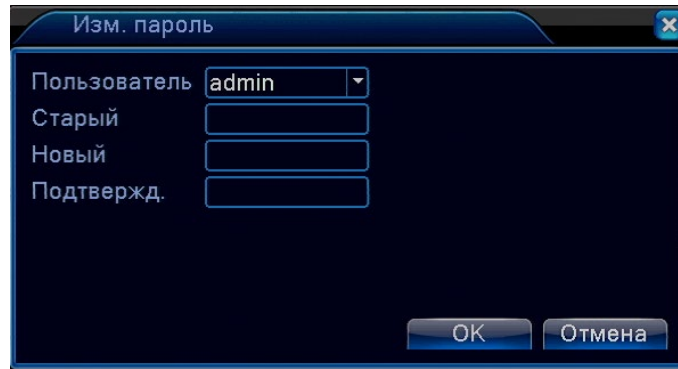
Рис. 4.29 Изменение пароля
