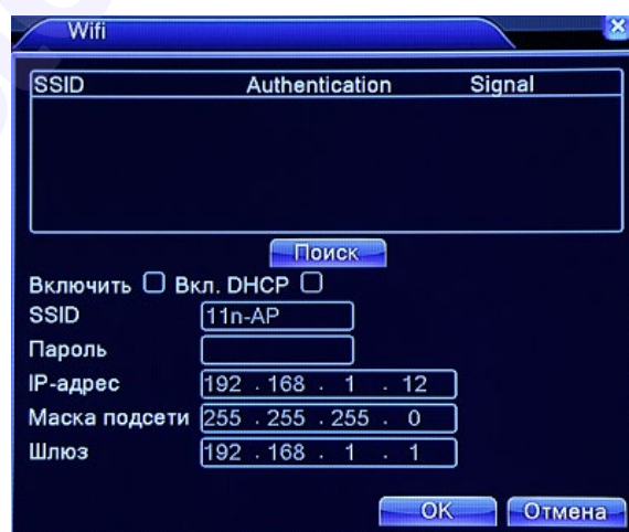
Рис. 4.15 Настройка Wi-Fi
