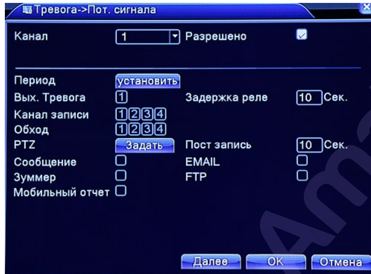
Рис 4.48 Потеря видеосигнала
