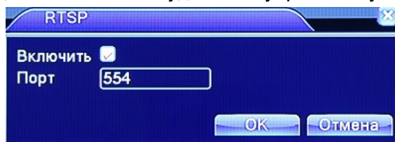
Рис. 4.16 Настройка RTSP
