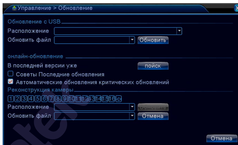
Рис. 4.62 Обновление ПО
