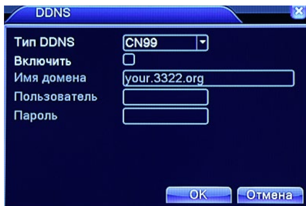
Рис. 4.8 Установка DDNS
