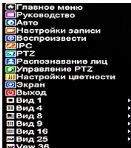
Рис 3.2 Контекстное меню
