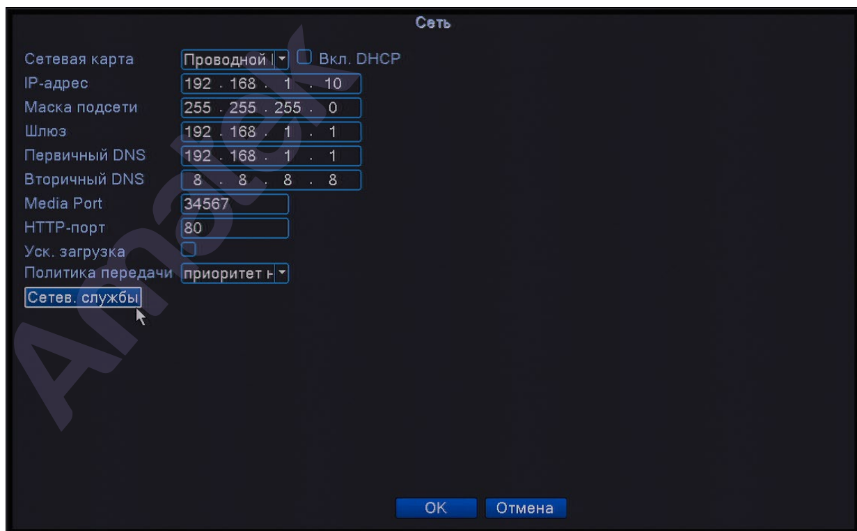
Рис. 4.2 Сетевые настройки
