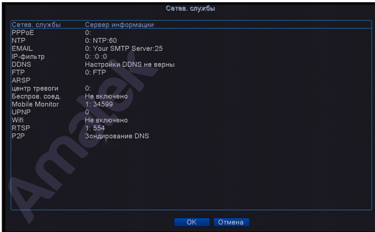
Рис. 4.3 Сетевые службы
