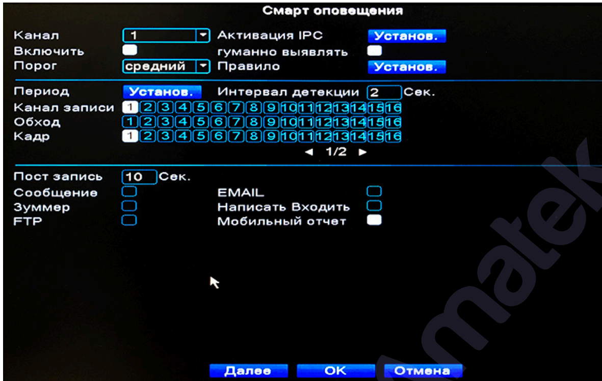
Рис 4.43 Смарт оповещения
