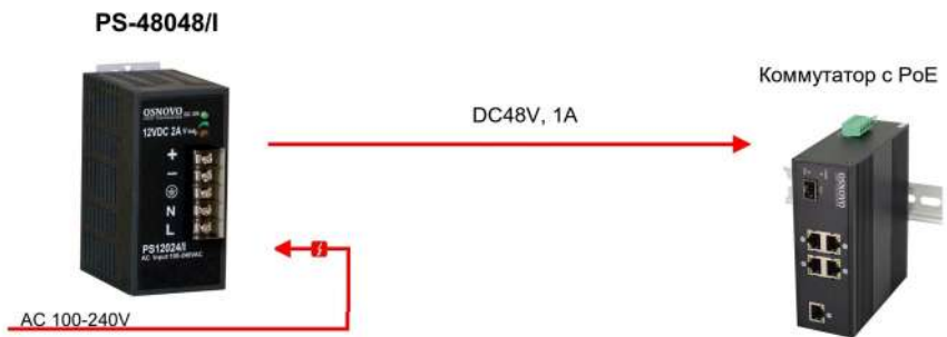
Рис. 5 Подключение PS-48048/I
